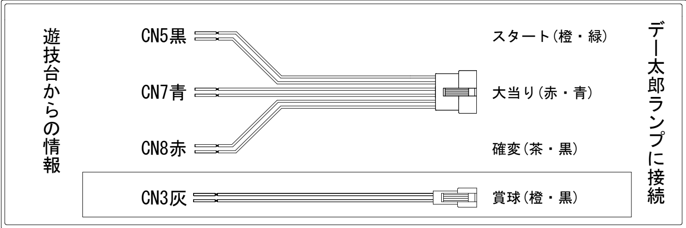
外部端子板
