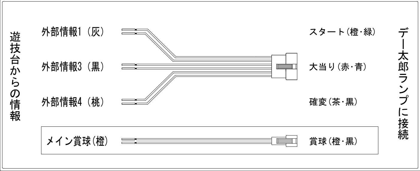
外部端子板
