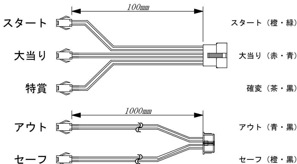
ハーネス結線図
