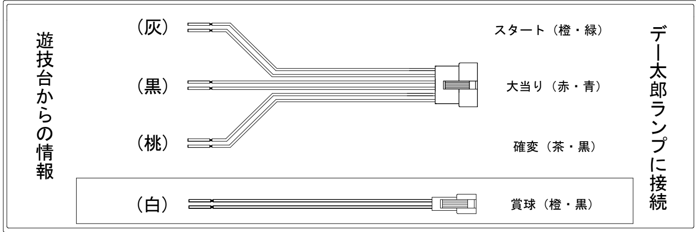
ハーネス結線図
