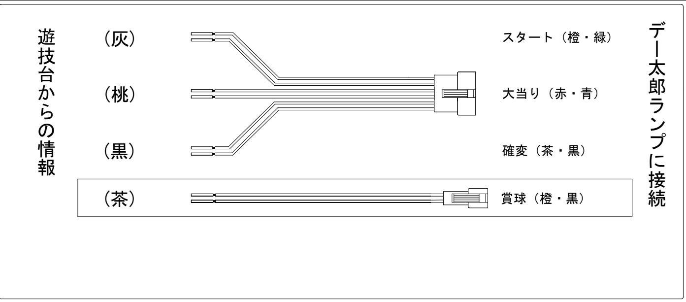
外部端子板
