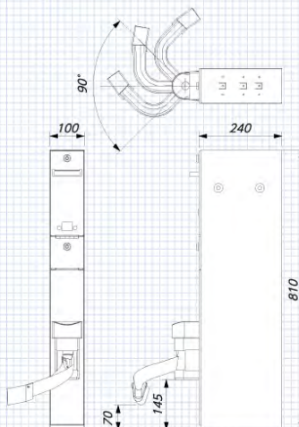
ノズルタイプ
