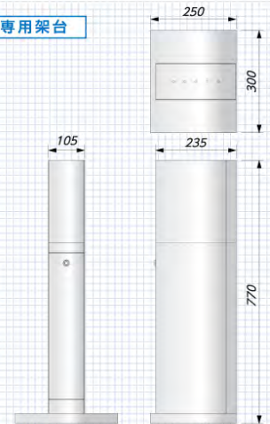
本体+専用架台
