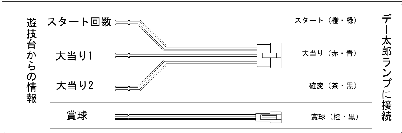
外部端子板
