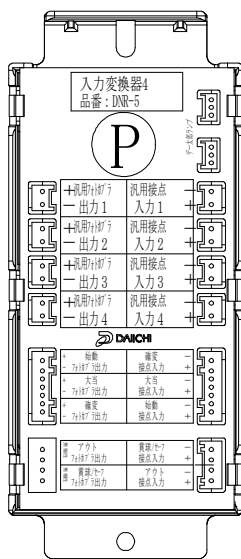
入力変換器 DNR-5
